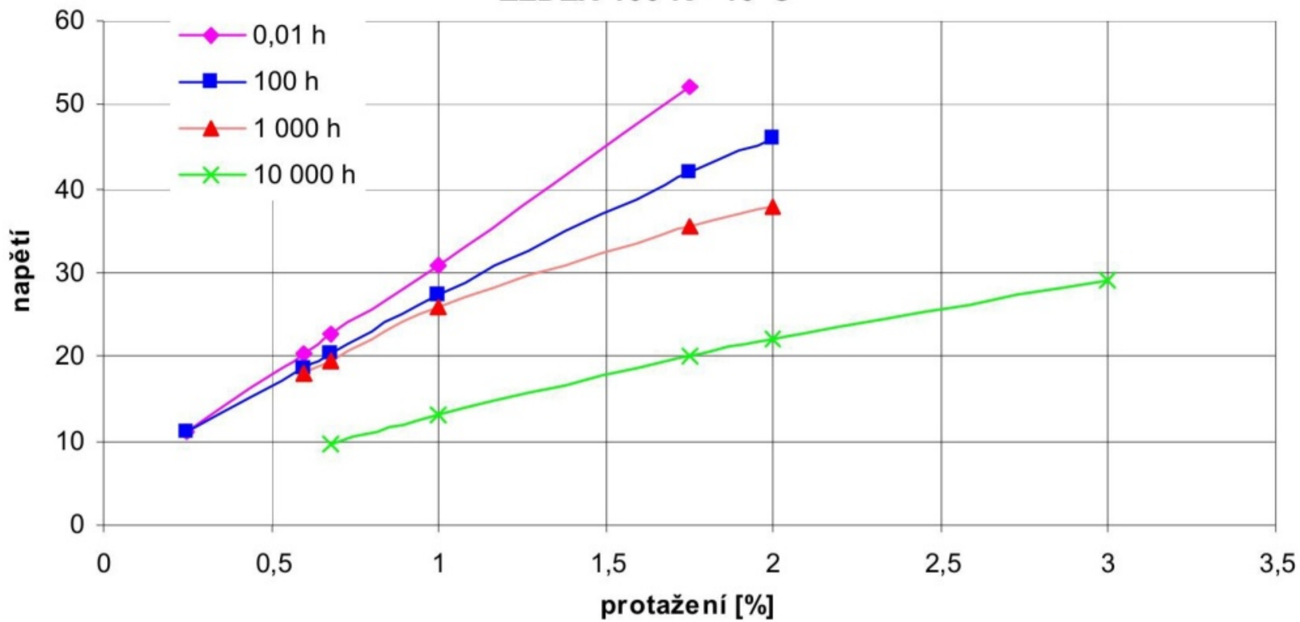
ZEDEX 100 K - 10°C
